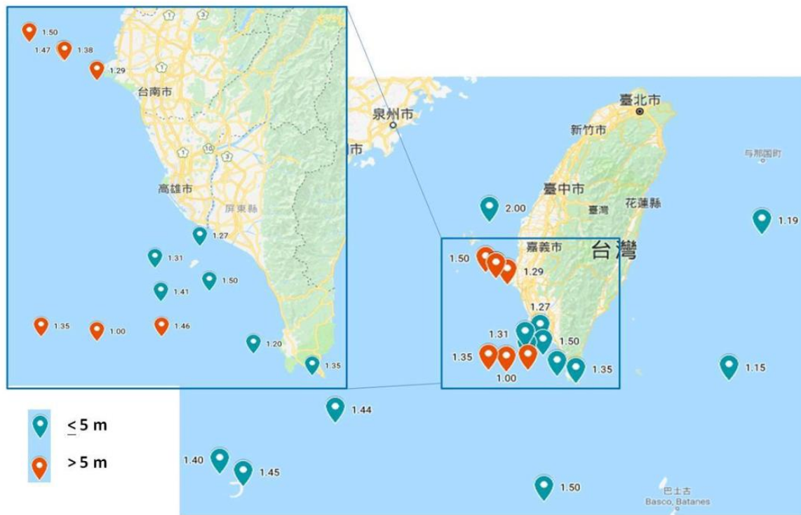
圖2 跨部會離岸海水取樣點及銫-137分析結果
