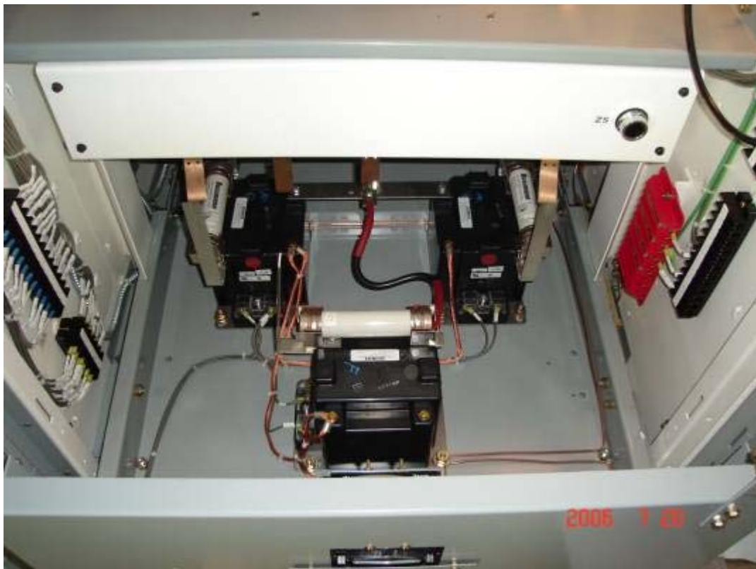
照片五：4.16kV 裝甲開關箱隔離板無法動作
